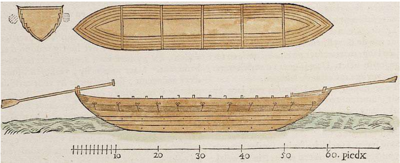
Козацька чайка. Креслення XVII ст.
