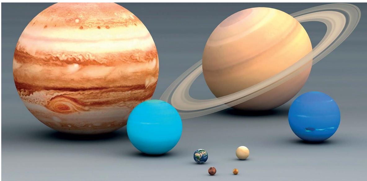
Юпітер, Сатурн, Уран, Нептун, Земля, Венера, Марс, Меркурій (у порядку зменшення розмірів)
